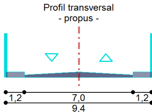
Profil transversal propus în zona accesului din Str. Profesor Alexe Marin
